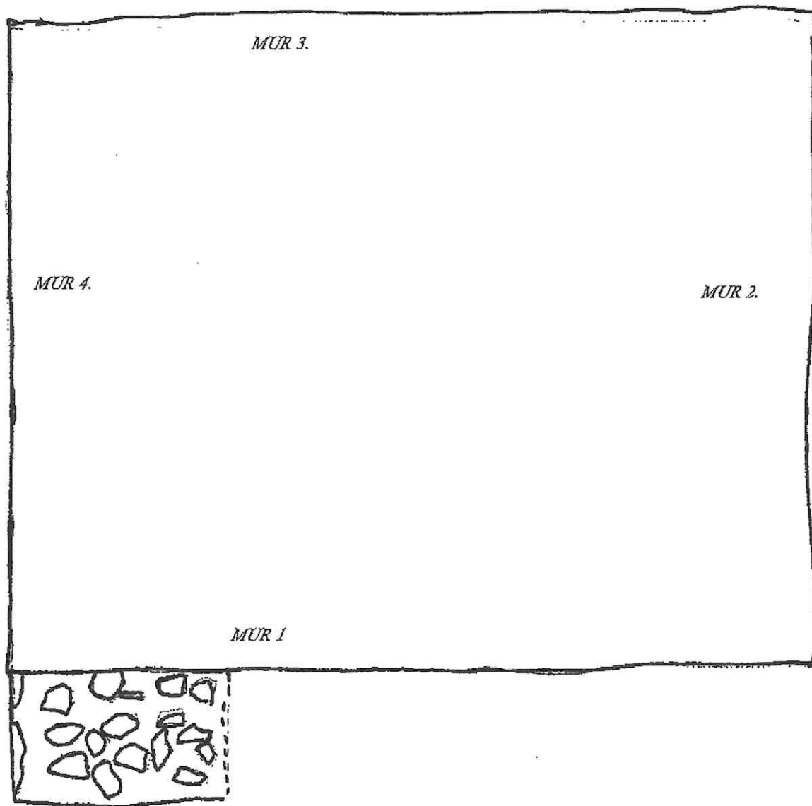
LA VINATERIA. PLANTA ESTRUCTURA. esc. 1/20
