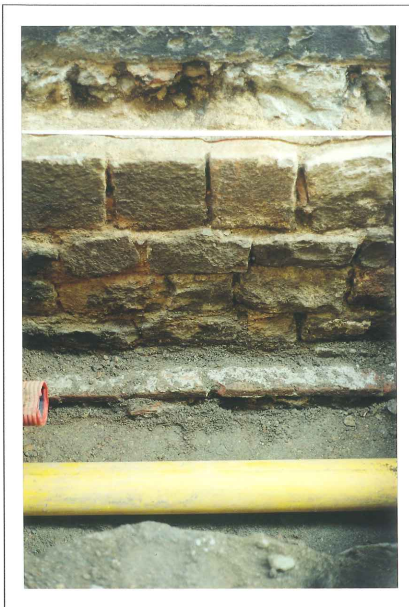
FOTO 2. Detall de la fonamentació descoberta durant l'obertura de la cala a la façana oest de l'església.
