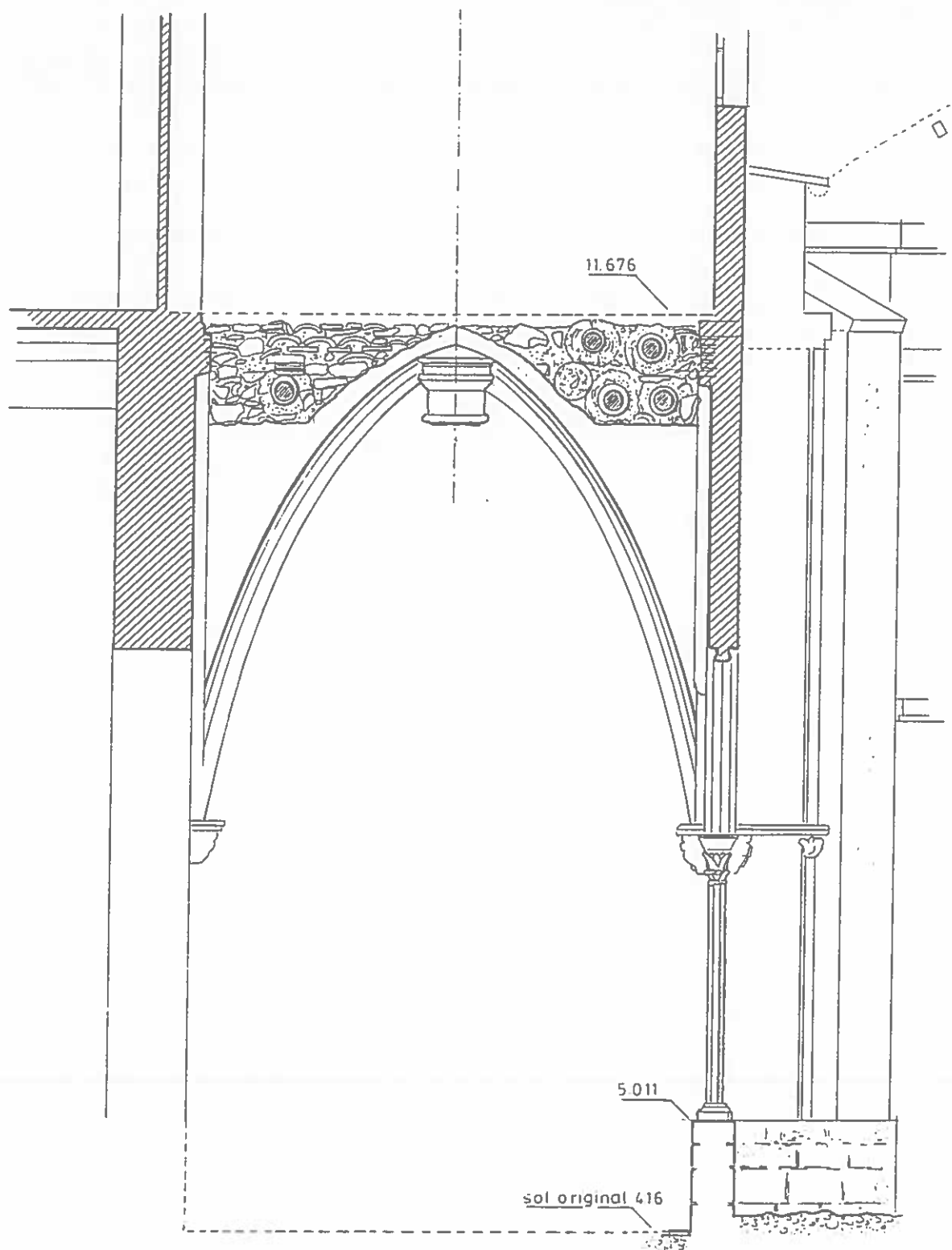
Secció transversal volta galeria
