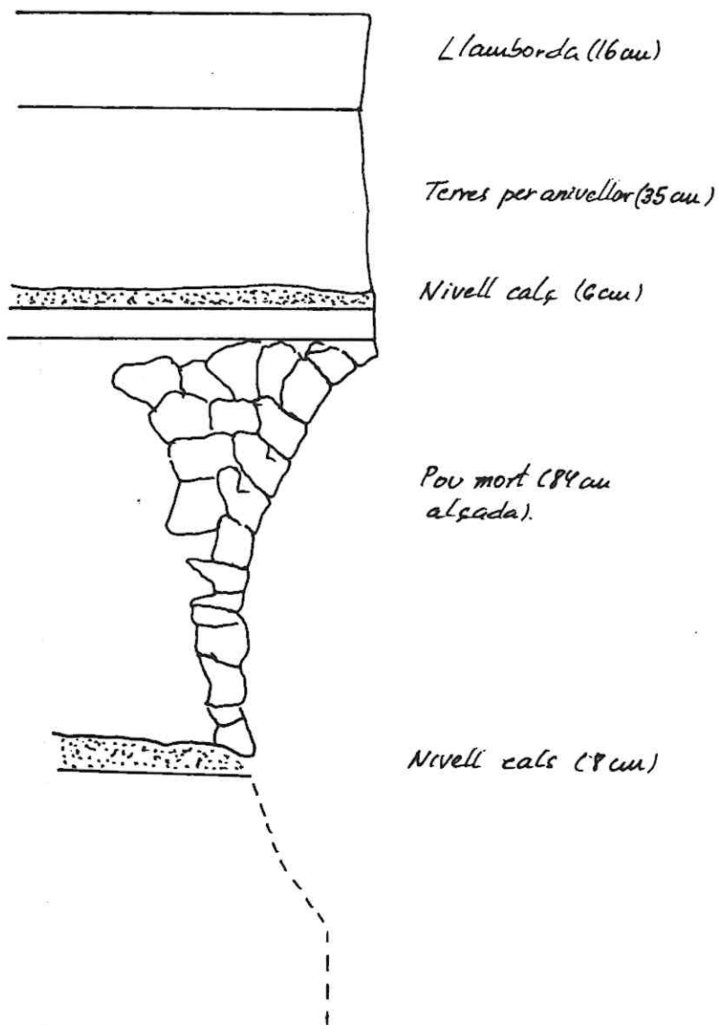
SECCIÓ PARET E. SECCIÓ POU MORT. (sense escala)
