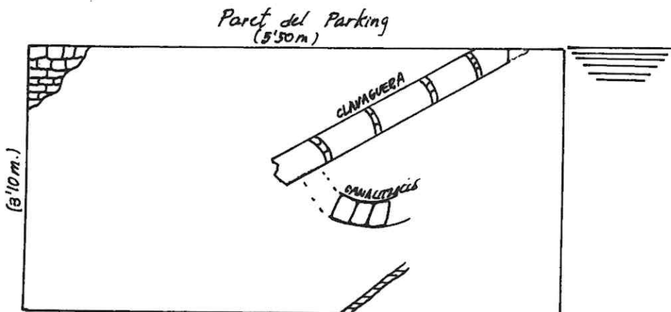
Planta - Croquis de l'Excavació amb les conduccions aparegudes a 60 cm. terra.
