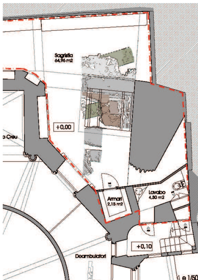
Fig.2 Planta de la sagristia amb la incorporació de la piscina baptismal com a element museïtzat i la recuperació del contrafort gòtic. Projecte Executiu: Figuerola Gavalda Romera arquitectes
