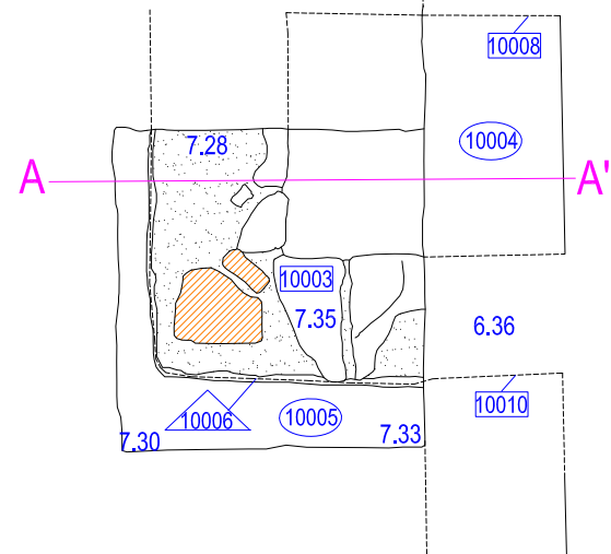
Planta 2
