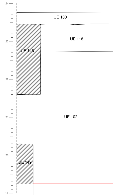
Secció D-D'
