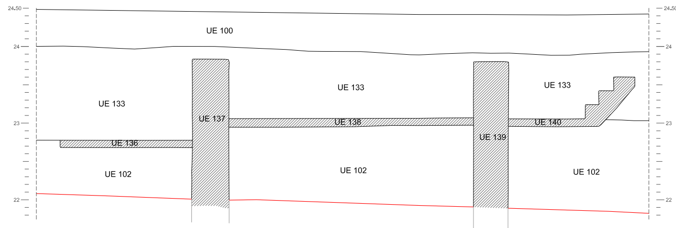
Secció C-C'
