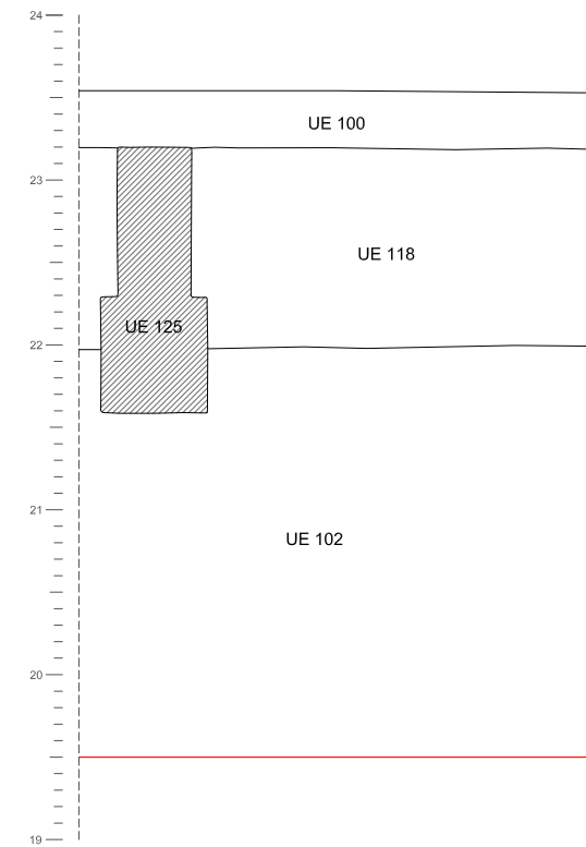
Secció E-E''
