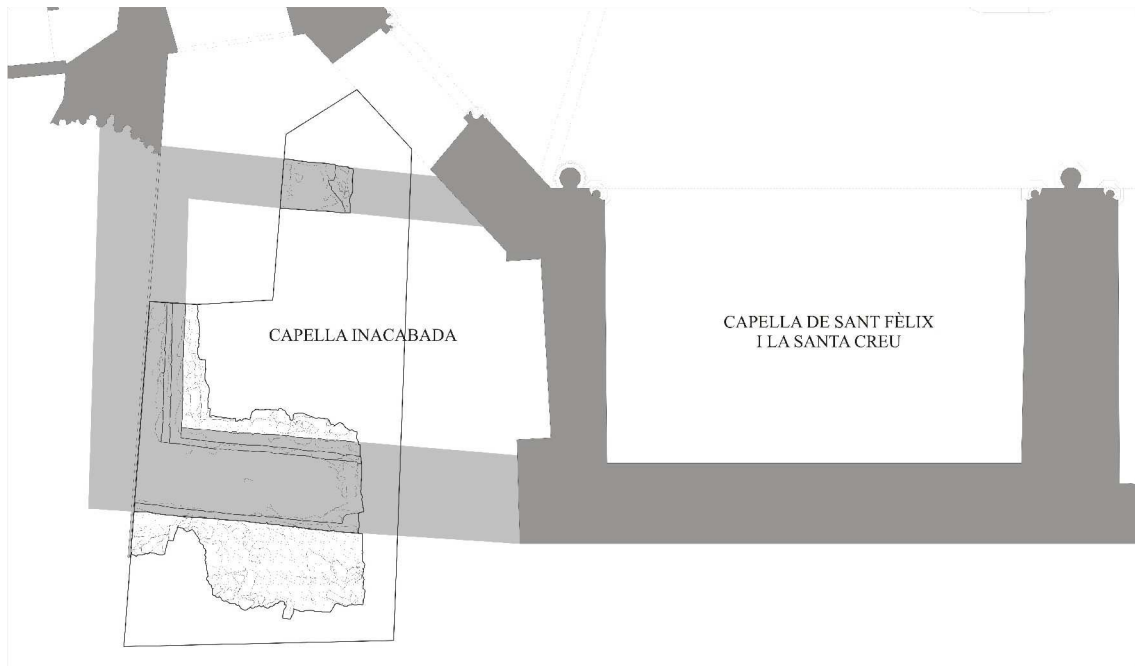
Fig.40 Planta de la capella gòtica inacabada (Ignasi Camps)
