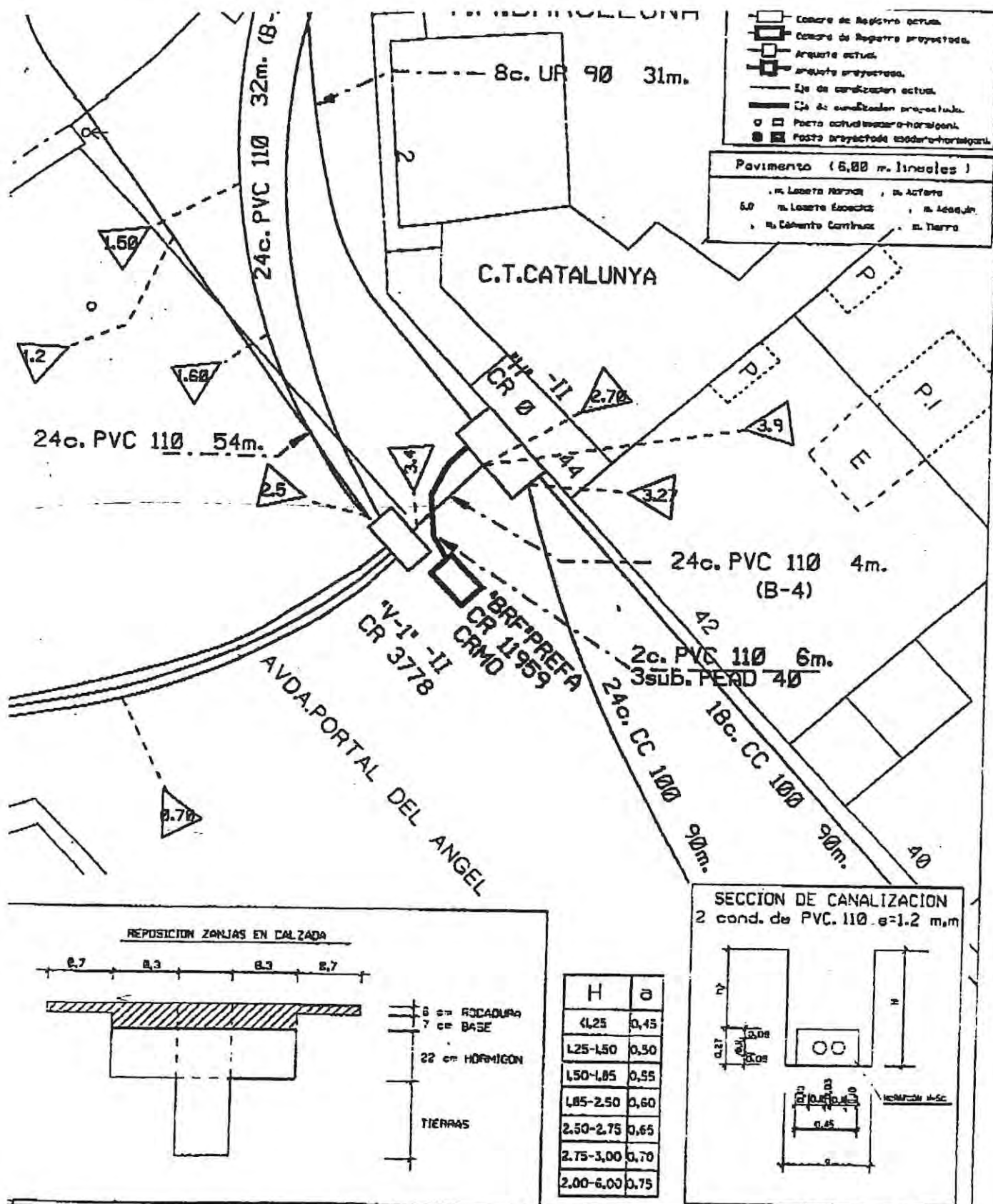
Figura 2. Projecte d'instal·lació de l'arqueta
